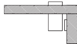
●外開き③ ストライク 埋込型
