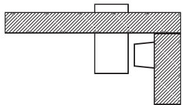
●外開き① ストライク 取付方法:L型
