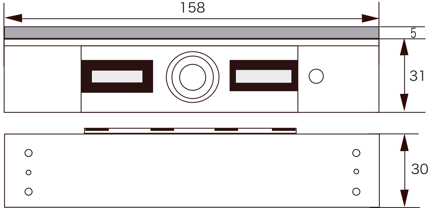
LC-MEM2400LP 本体 158×31×30 単位 mm
